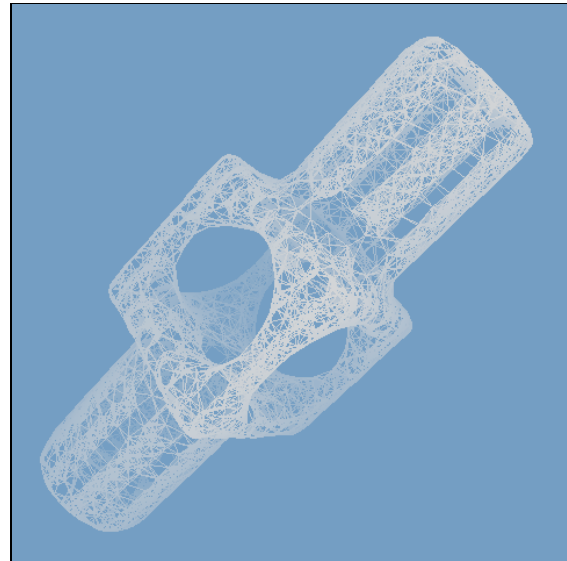
(d) Riemannian Graph over o_i
